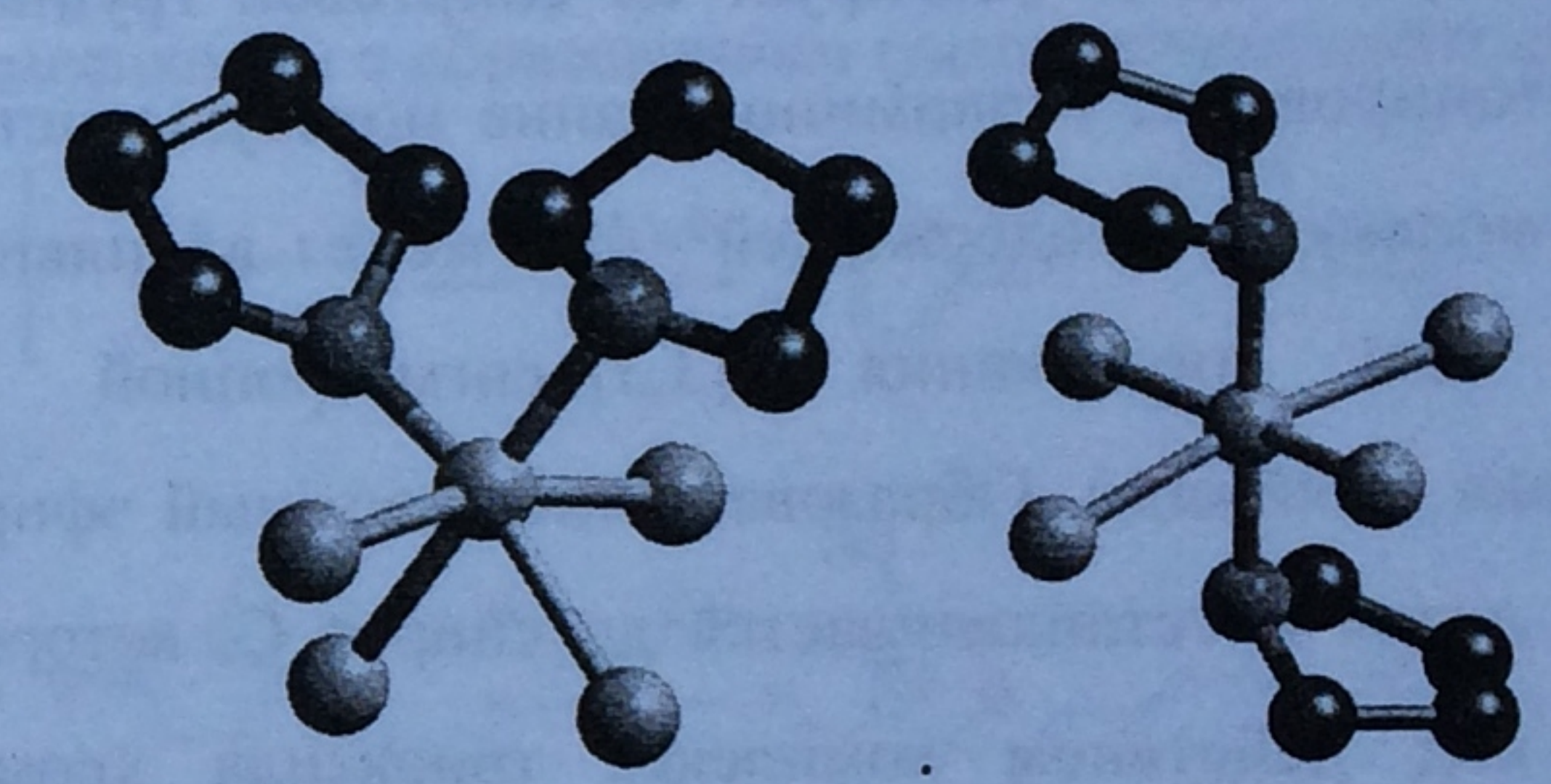
цис - [\text{TcCl}_4(\text{TГФ})_2]
