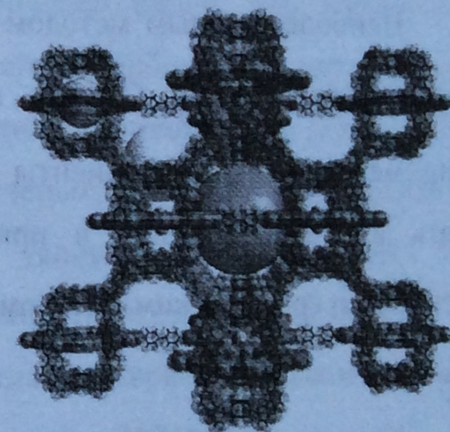
Строение DUT-49
